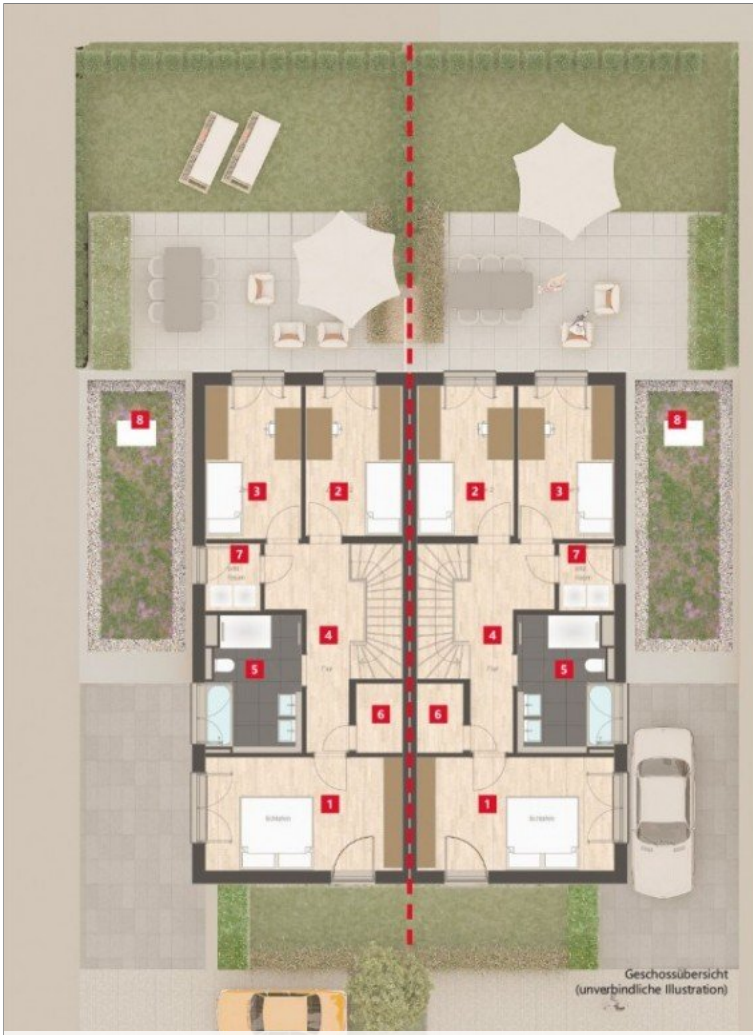
Grundriss Obergeschoss
